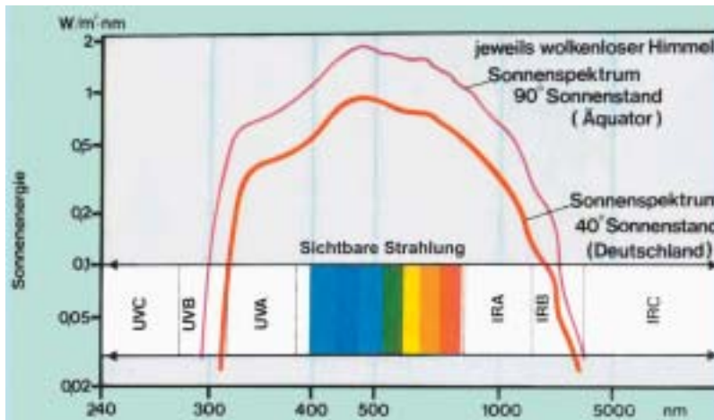
Abb. 9: Sonnenstrahlung auf die Erdoberfläche (schematisch)
